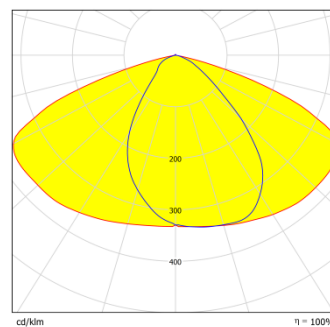
Lens Type TIII / Soczewka Typ TIII
