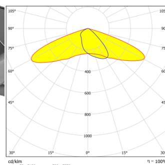
Lens Type TII / Soczewka Typ TII
