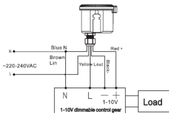
Wiring / Okablowanie
